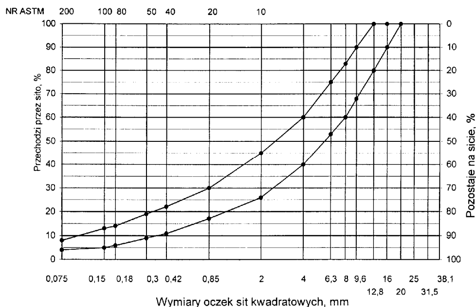
Rys. Krzywe graniczne uziarnienia mieszanki mineralnej BA od 0 do 16 mm do podbudowy nawierzchni drogi o obciążeniu ruchem KR 1 lub KR 2
